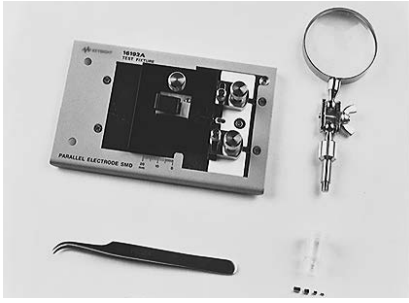
16192A 병렬 전극 SMD 테스트 픽스처
